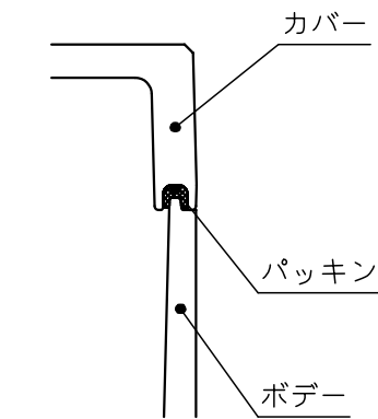
水切部断面図 (1/1)
