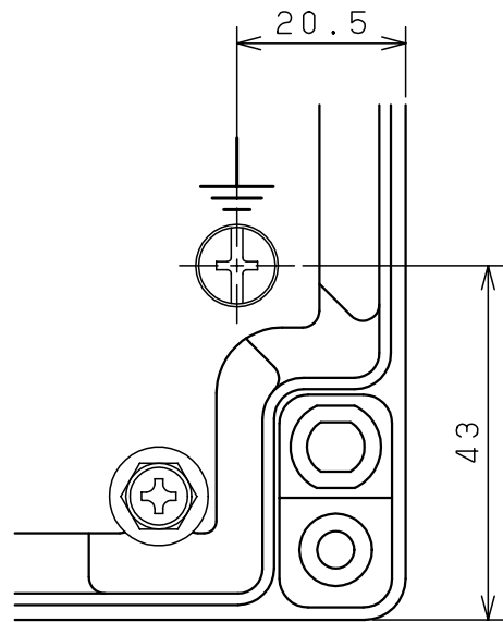
アース部詳細 (1/1)
