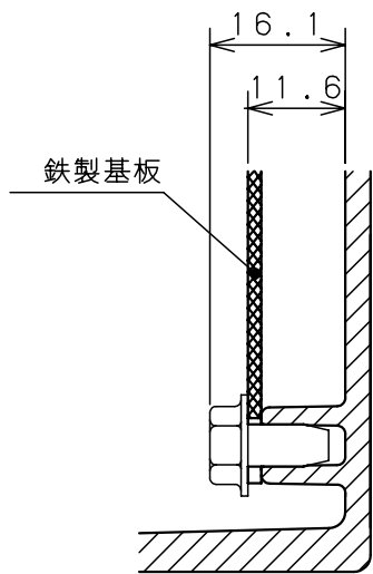
基板断面図 (1/1)
