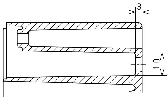
A-A断面
