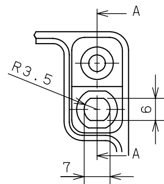
ボックス取付穴詳細
