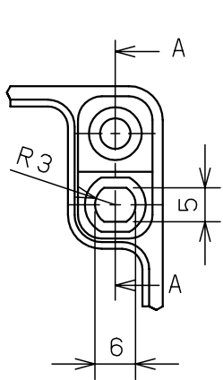
ボックス取付穴詳細
