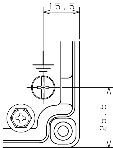
アース部詳細 (1/1)
