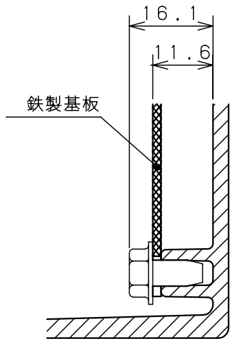
基板断面図 (1/1)
