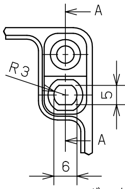
ボックス取付穴詳細
