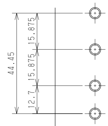
A部詳細 (1 : 1)
