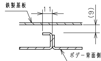
F-F断面詳細
