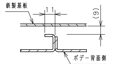
F-F断面詳細
