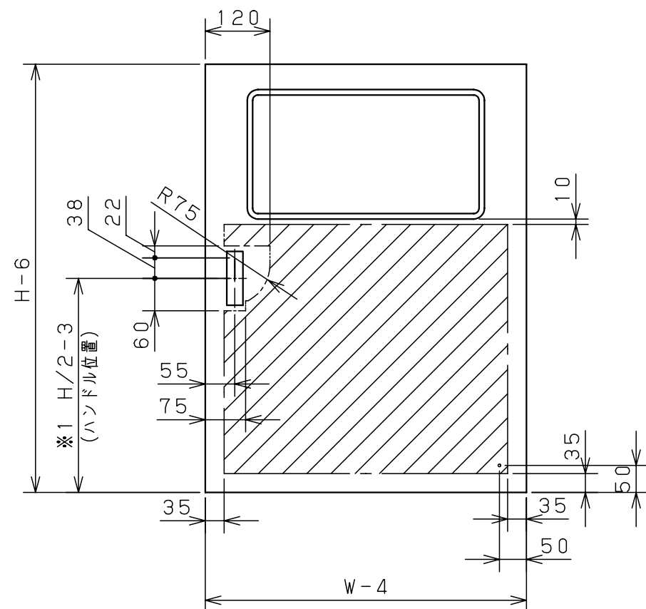
扉 機器取付有効図
