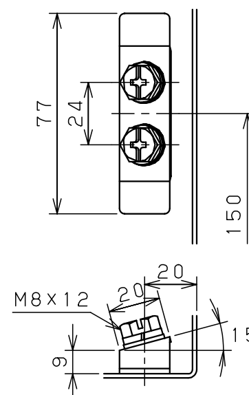
C部接地端子詳細 (1 : 2) (国土交通省仕様)
