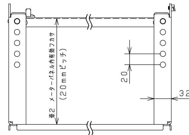
メーターパネル図
