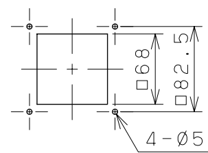
取付穴寸法
