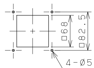
取付穴寸法
