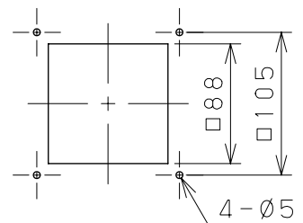
取付穴寸法
