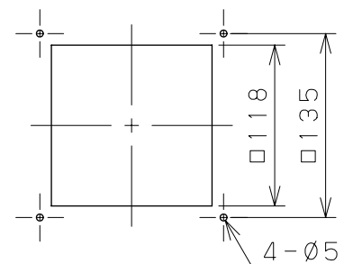
取付穴寸法
