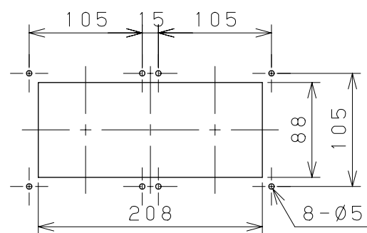
取付穴寸法
