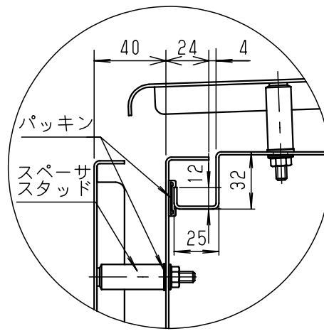
A部断面詳細 (1:3)
