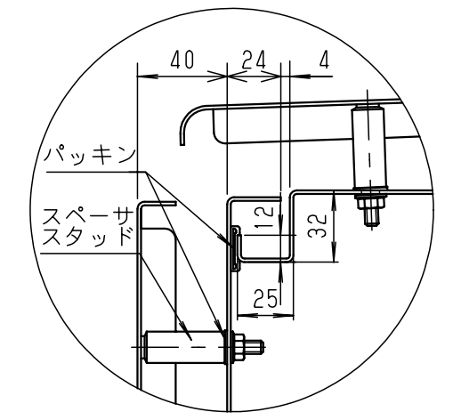
A部断面詳細 (1:3)
