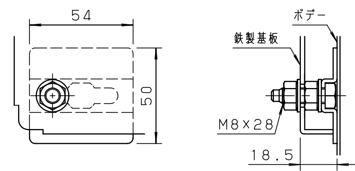
基板取付部詳細 (1:2)
