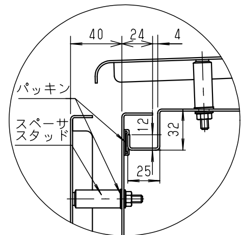
A部断面詳細 (1:3)
